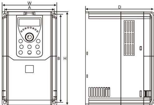
图6-2 外型尺寸及安装尺寸示意图
